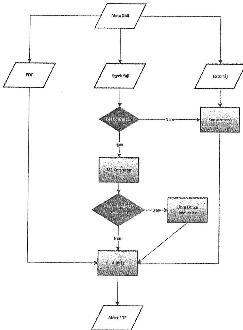
3. ábra – Az RZS Signer rendszerszintű működése
