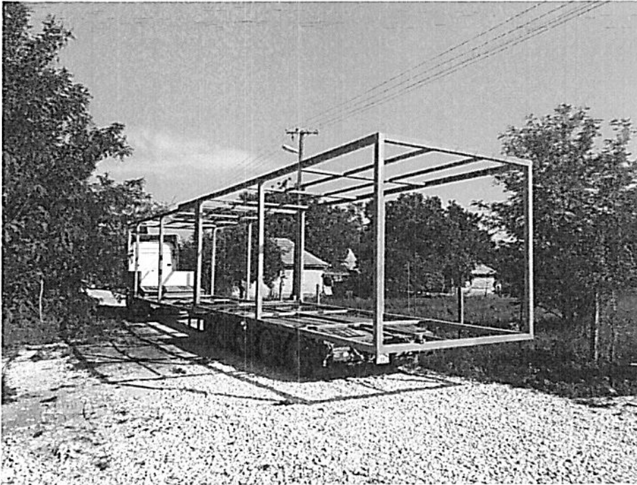
Kép: PuzzleHome mobilház alvázszerkezete
